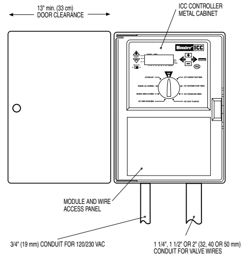
Hunter® ICC-M
