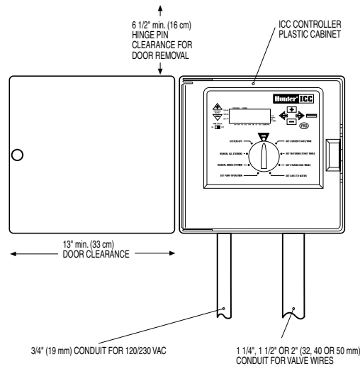
Hunter® ICC-PL
